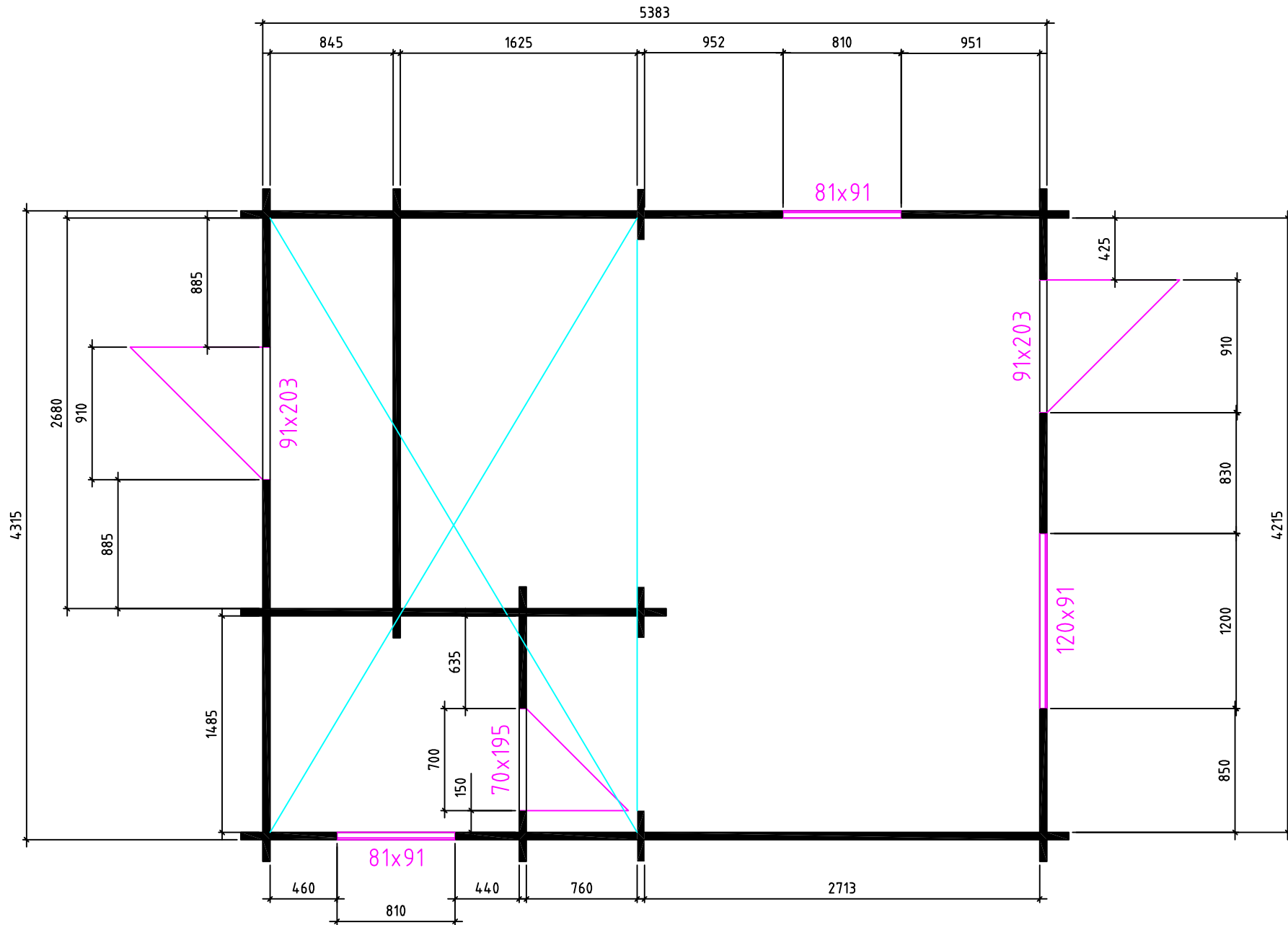
Grundplan
