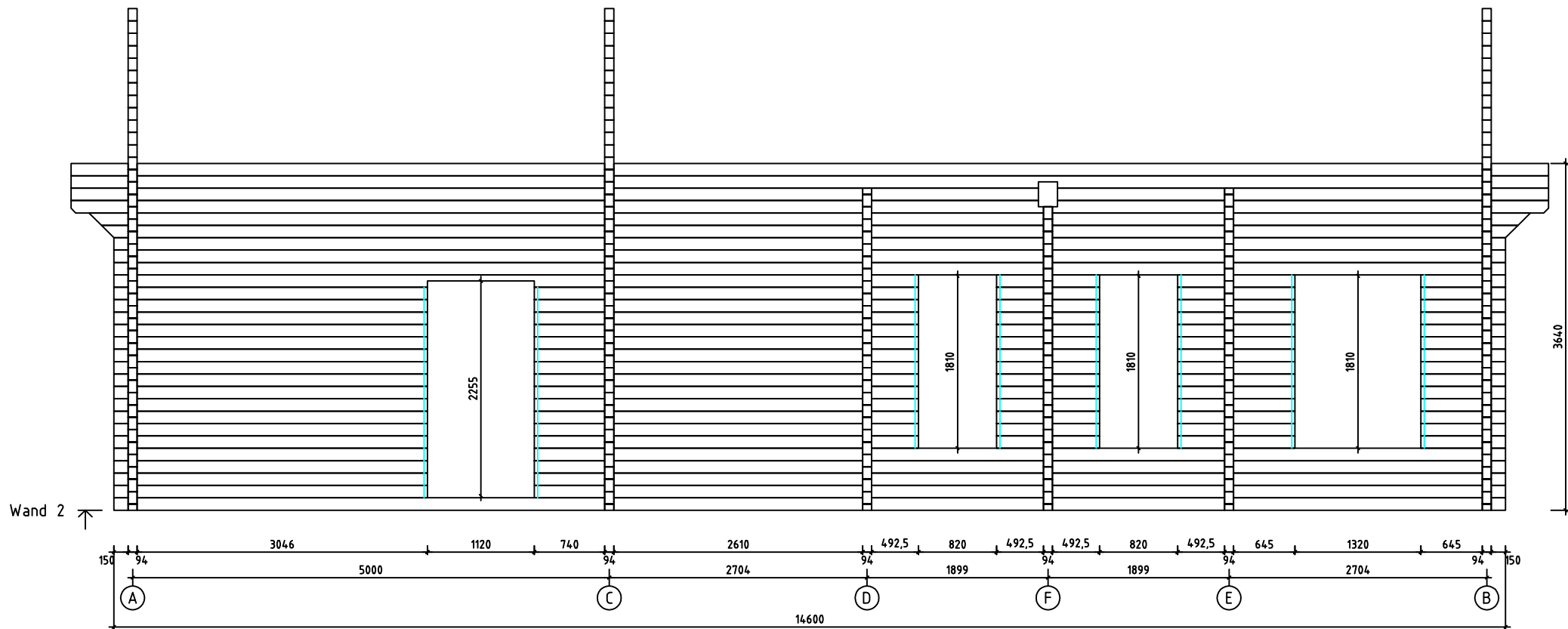
Haus 9000x14300 / 94 / 12 /
