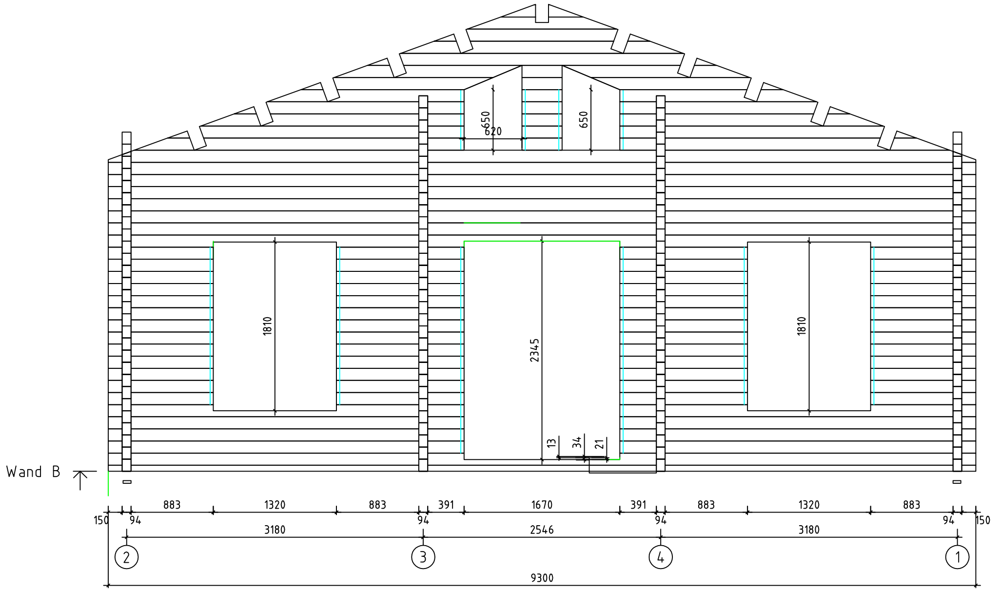
Haus 9000x14300 / 94 / 12 /
