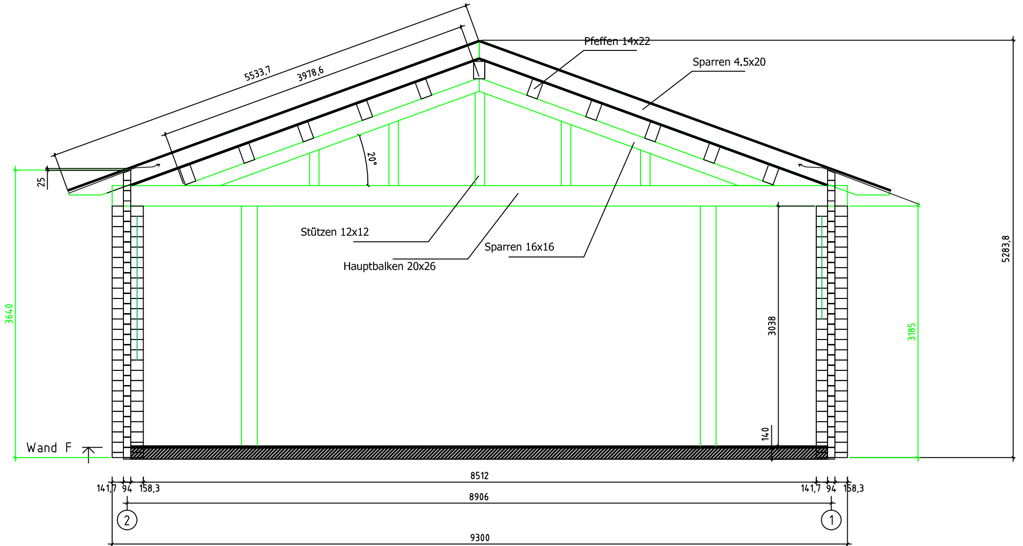
Haus 9000x14300 / 94 / 12 /
